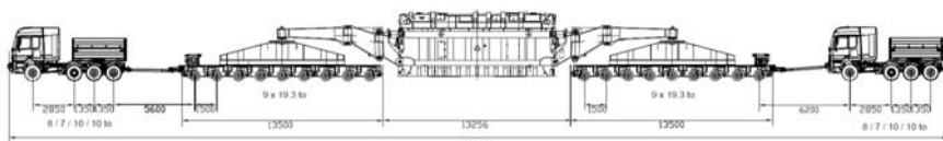
Convoi de 310 t par l'entreprise Felbermayr
