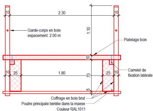
Coupe type
